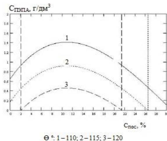
Рис. 2. Двухфакторная номограмма: \theta=f(C_{\text{ПЭПА}}, C_{\text{ПФС}}) при T=25^\circ\text{C} для алюминиевой подложки
