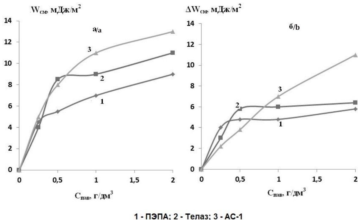
Рис. 1. Влияние поверхностно-активных веществ на изменение работы смачивания ( \Delta W_{\text{см}} ) в отношении алюминия (а) и стали (б) (содержание полифенилсилоксанов 30 % (по массе)) при t=25^\circ\text{C}
