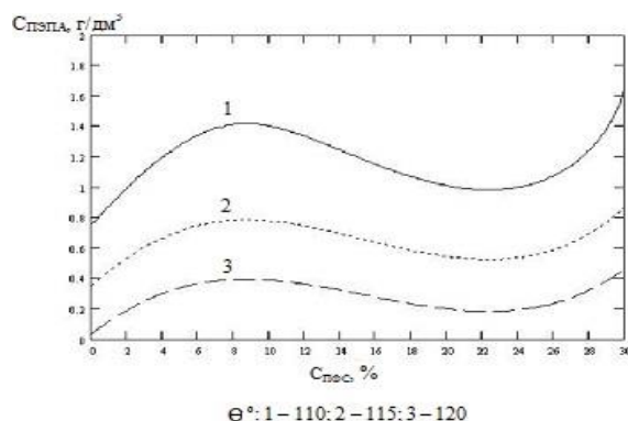
Рис. 3. Двухфакторная номограмма: \theta = f(C_{\text{СППА}}, C_{\text{ППС}}) ; при T = 25^\circ\text{C} для стальной подложки
